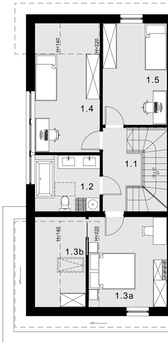
RZUT PIĘTRA
